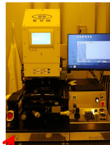
Mask Aligner EVG620 NT
